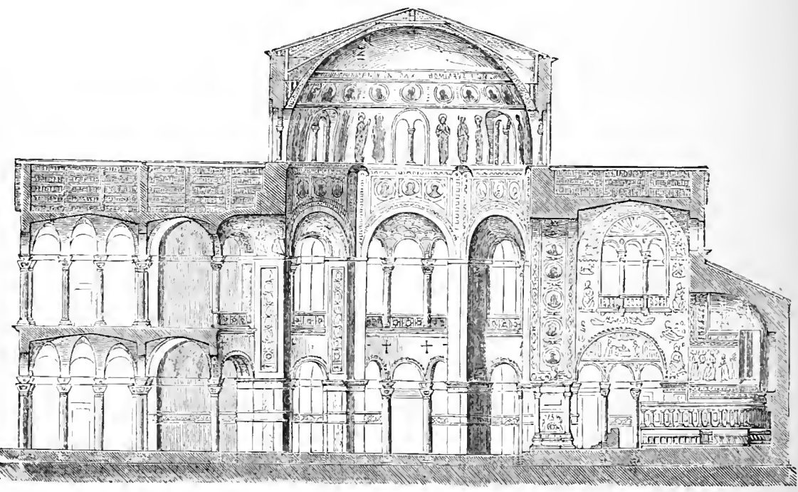
FIG. 161.—SAN VITALE AT RAVENNA. LONGITUDINAL SECTION
